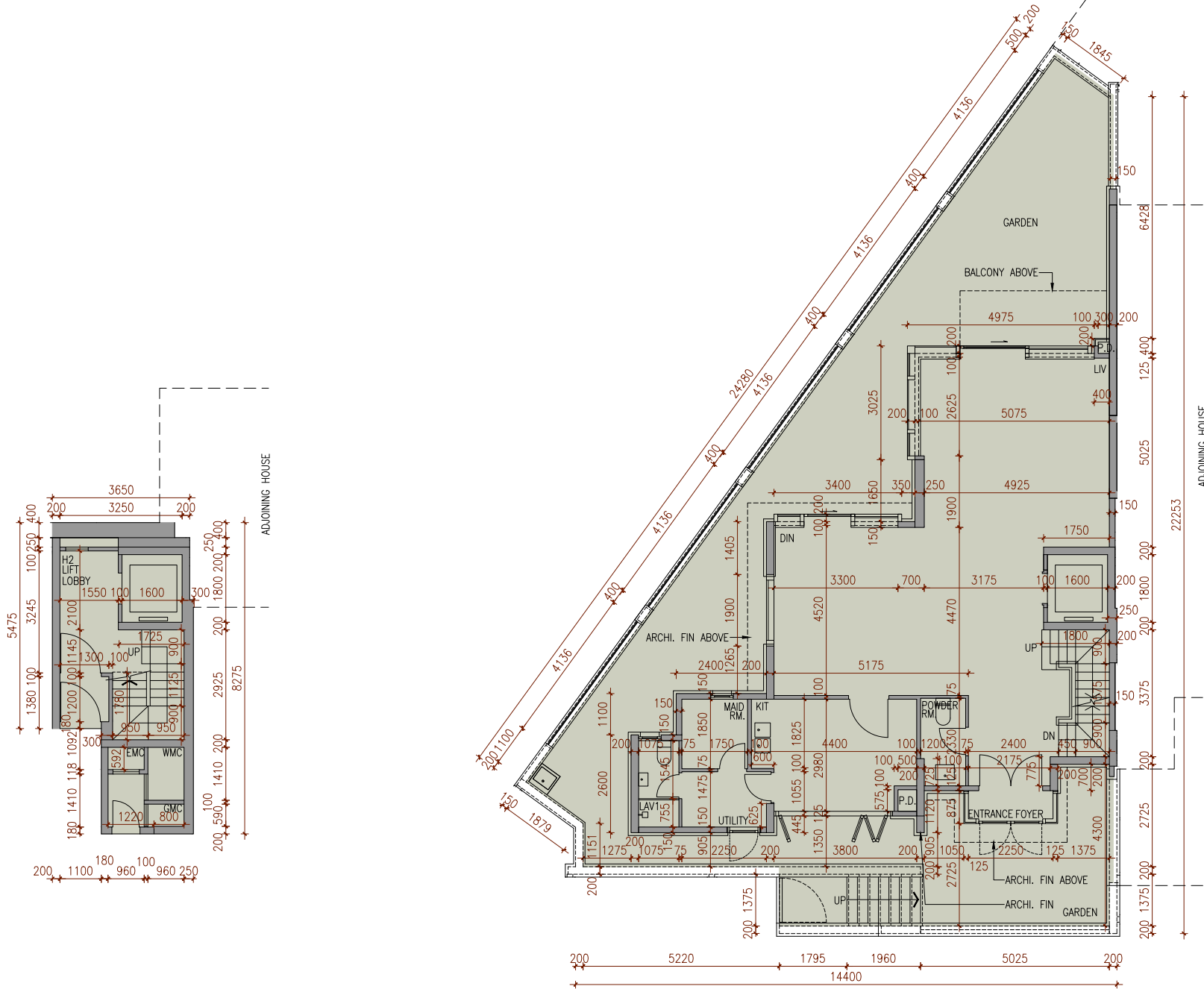
BASEMENT FLOOR PLAN 地庫層平面圖
