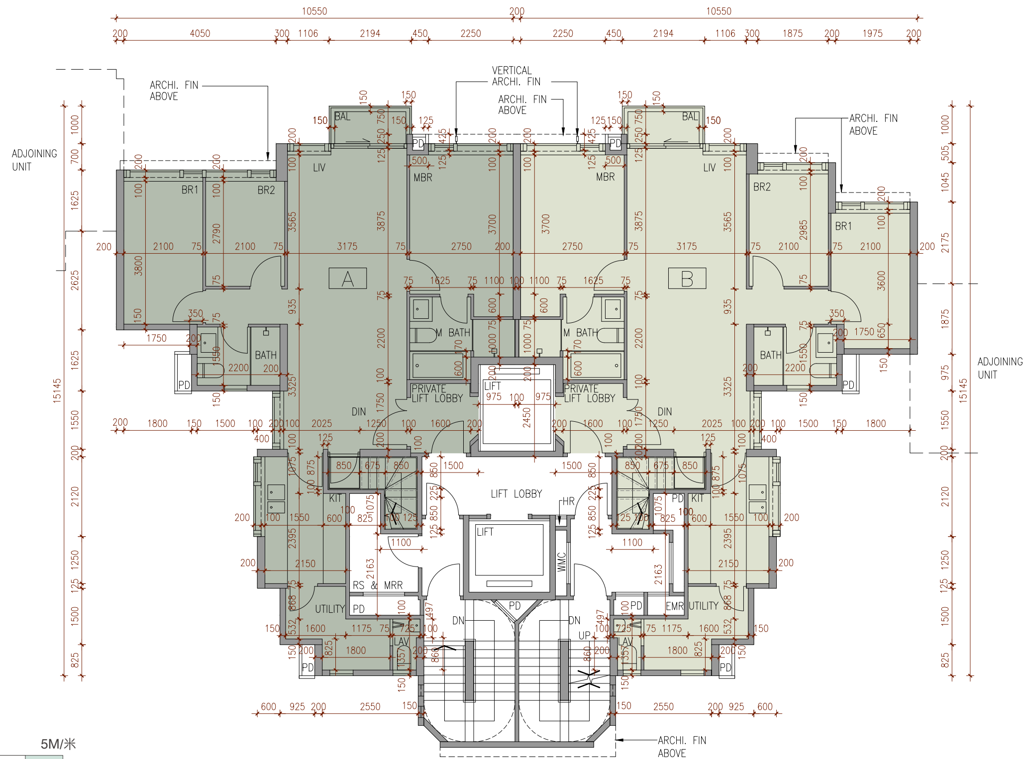
TOWER 2 第2座 15/F FLOOR PLAN 15樓平面圖
