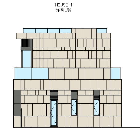
ELEVATION PLAN 4 立面圖 4
